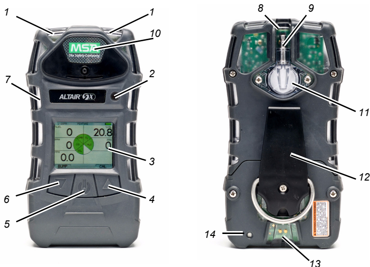
Bild 1 Ansicht des Geräts
